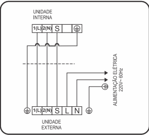
Esquema de ligação de unidades Cassete modelos 24/30.000 - 220V ~ (Quente/Frio)
