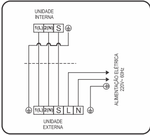
Esquema de ligação de unidades Piso-Teto modelos 24/30.000 - 220V ~ (Quente/Frio)
