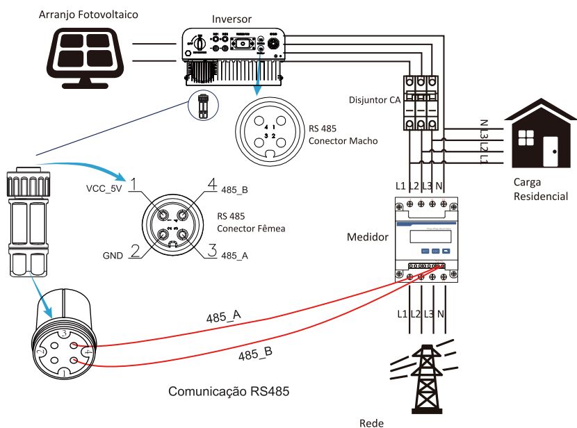
Figura 7.16 Conexão do diagrama do medidor CHINT
