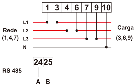
Figura 7.15 Medidor CHINT
