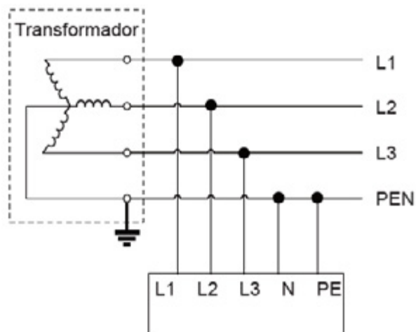
TN-C
