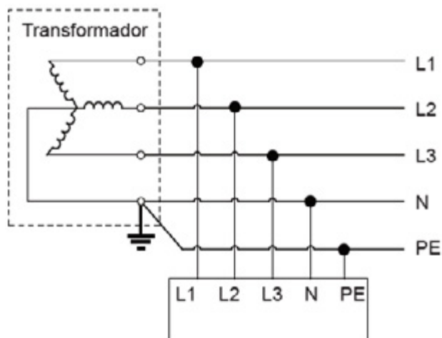
TN-S
