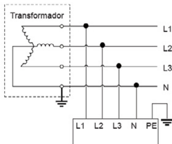
TT
