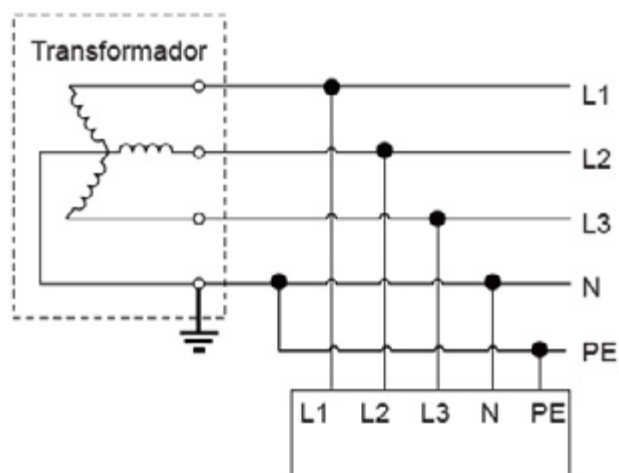
TN-C-S
