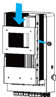
Instalação da placa suspensa do inversor
