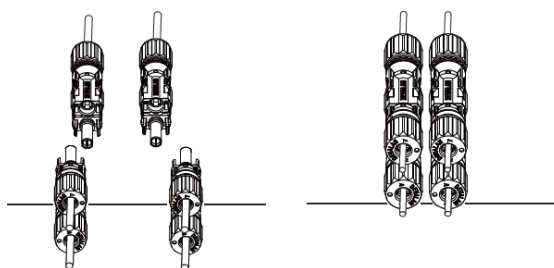
Figura 3.6 Conexão de entrada CC
