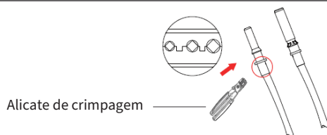
Figura 3.4 Prenda o pino de contato no fio
