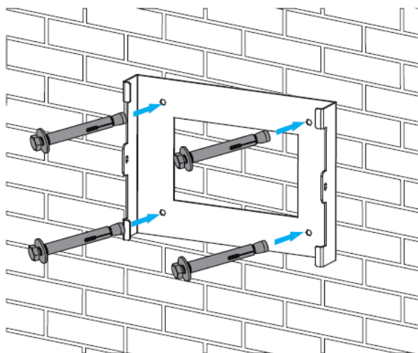
Instalação da placa suspensa do inversor
