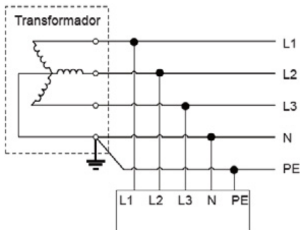
TN-S
