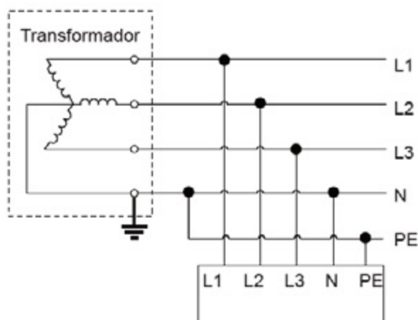
TN-C-S
