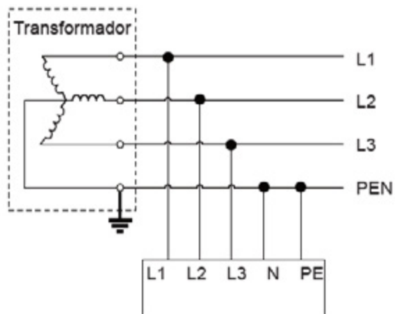
TN-C
