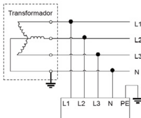
TT
