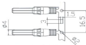
Contato do pino macho (-)
