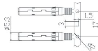
Contato do pino fêmea (+)
