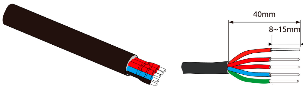
Figura 5.8 Desencapar o cabo AC
