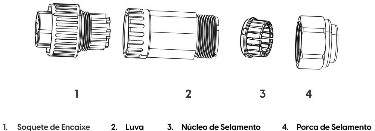
Figura 5.7 Estrutura do Conector CA
