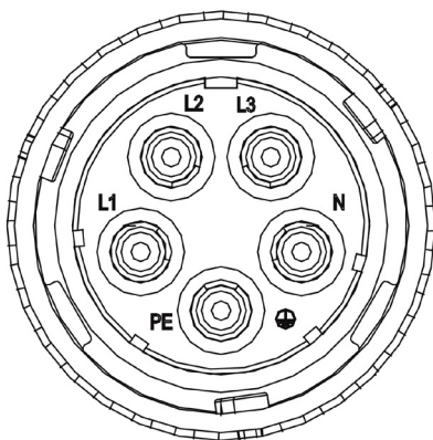
Figura 5.9 Padrão de furo do conector AC
