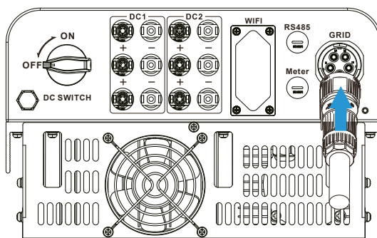
Figura 5.10 Conexão de entrada AC
