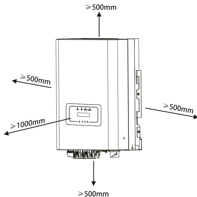
Figura 4.3 Espaçamento de Instalação
