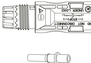
Figura 5.2 Conector DC- (MC4)
