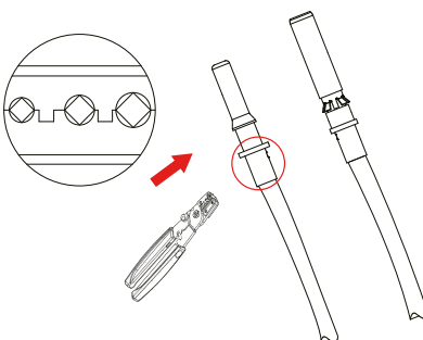
Figura 5.4 Crimpe o pino de contato no fio
