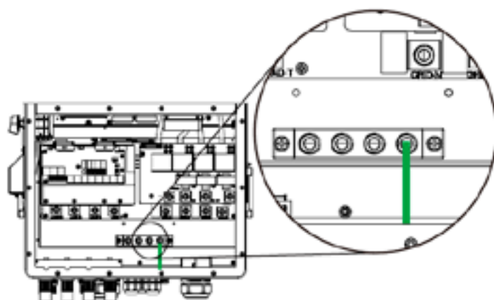
Conexão do aterramento (Condutores de cobre) (bypass)
