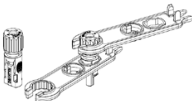
Figura 5.5 Conector com porca de capa parafusada
