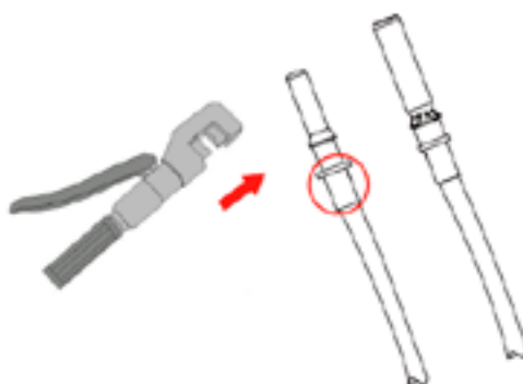
Figura 5.4 Crimpe o pino de contato ao fio
